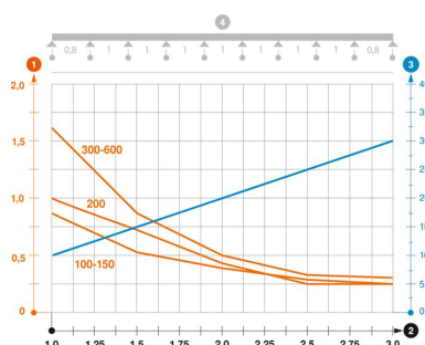
Belastingsdiagram draadgoot type GRM 105
